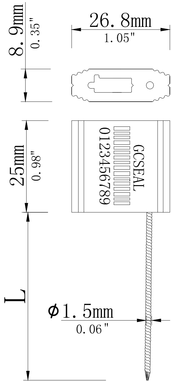
Model : GC-C1502
